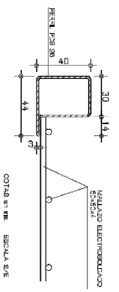
DETALLE MARCO PERIL PDS 28 Y MALLAZO
